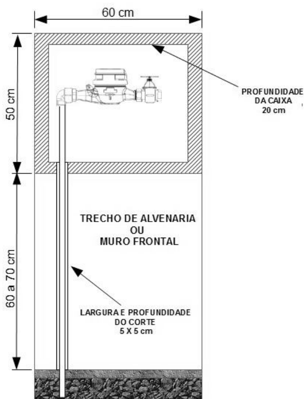
Fig 06. Modelo do abrigo protetor para ligação de água.
