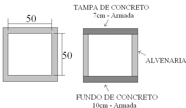
Fig 07. Modelo da caixa de inspeção para a ligação de esgoto.
